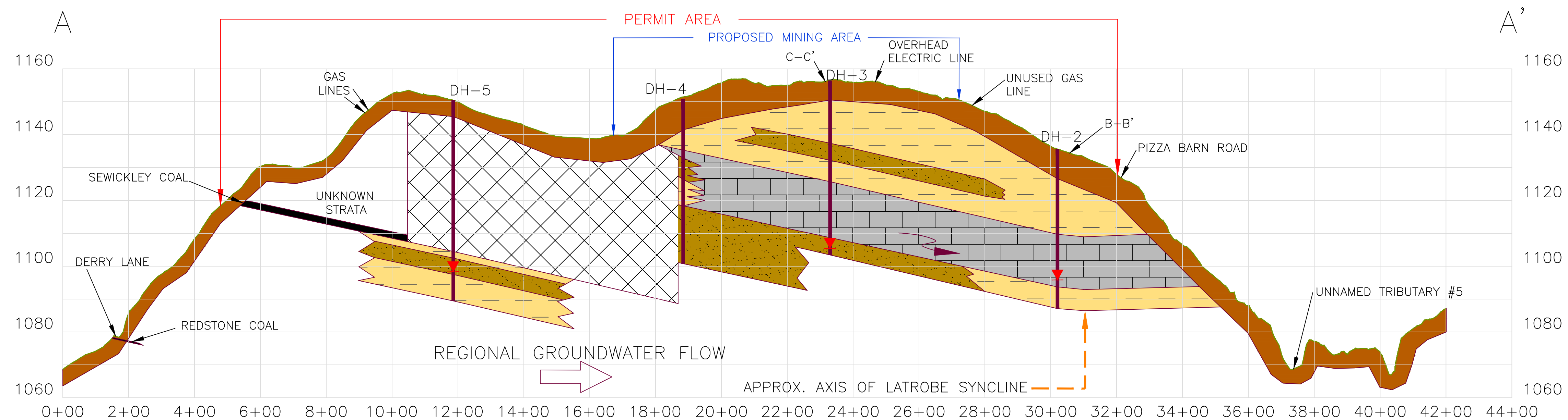
CROSS SECTION A-A' HORIZONTAL SCALE: 1" = 200' VERTICAL SCALE: 1" = 20'
