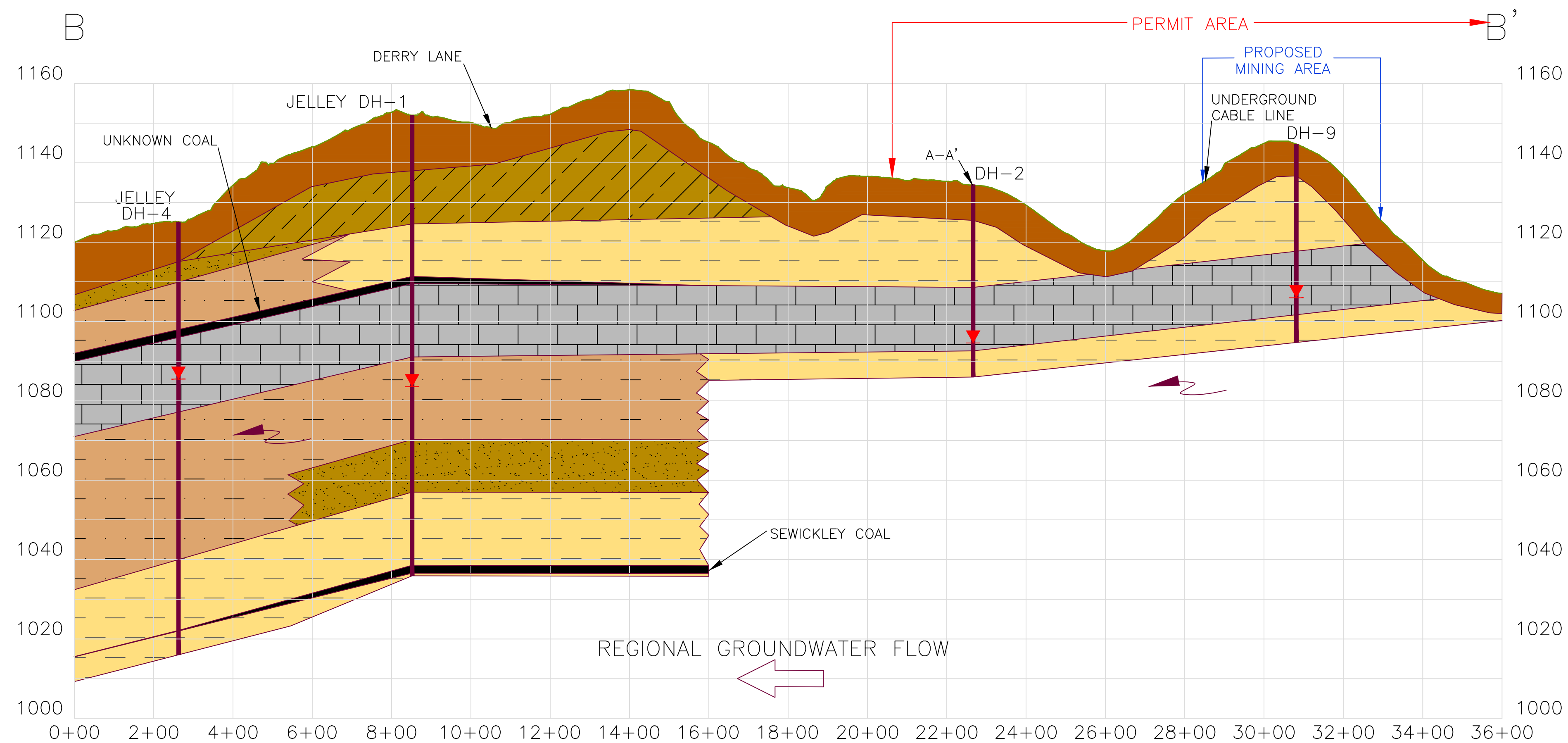
CROSS SECTION B-B' HORIZONTAL SCALE: 1" = 200' VERTICAL SCALE: 1" = 20'
