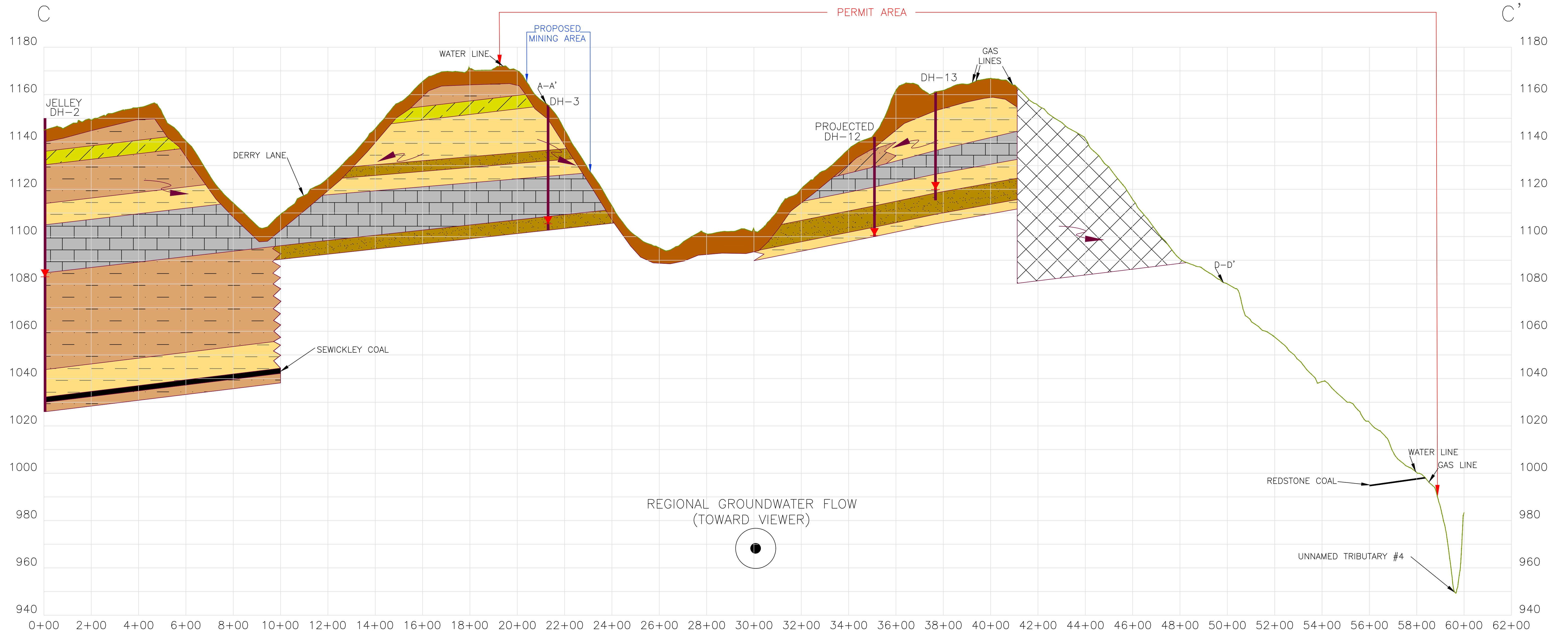
CROSS SECTION C-C' HORIZONTAL SCALE: 1" = 200' VERTICAL SCALE: 1" = 20'
